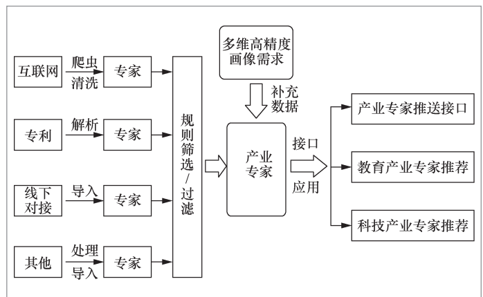
图2 专家数据集成系统架构
