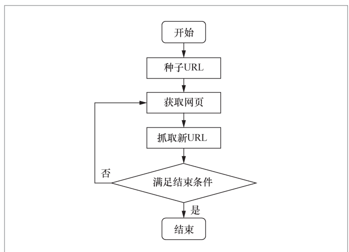
图3 爬虫流程
