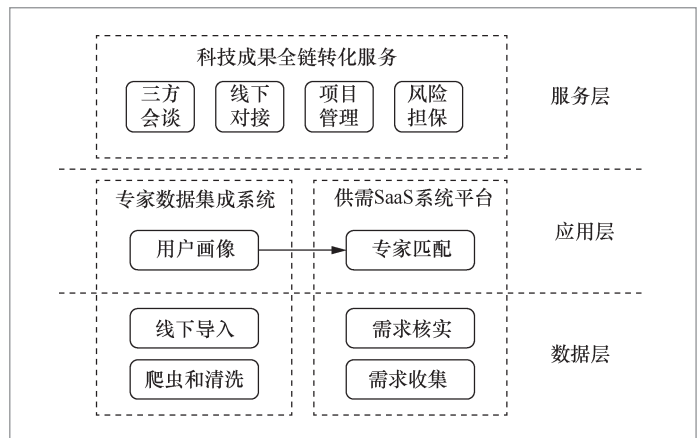
图1 系统整体架构
