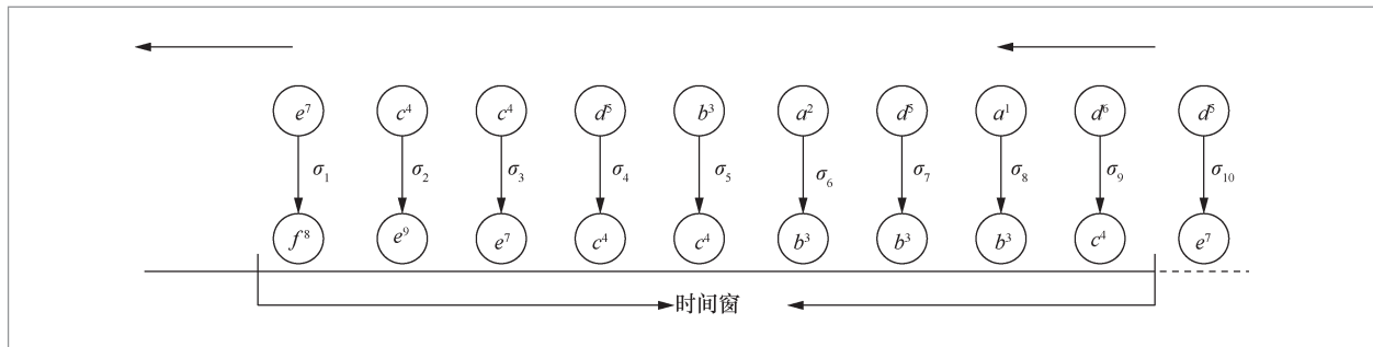
图2 带时间窗的图数据流示例
