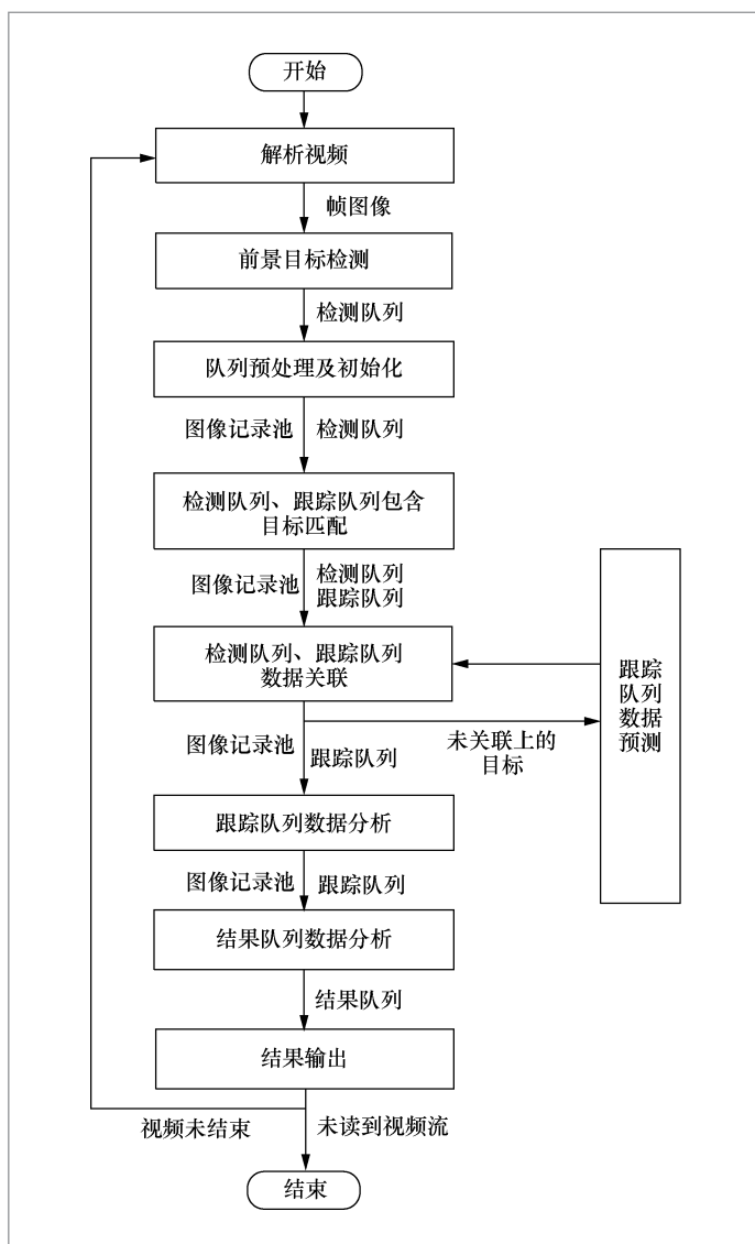
图6 视频内容挖掘流程
